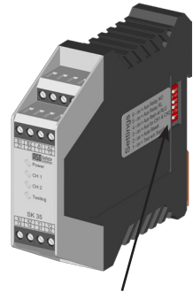
Commutateurs DIP
