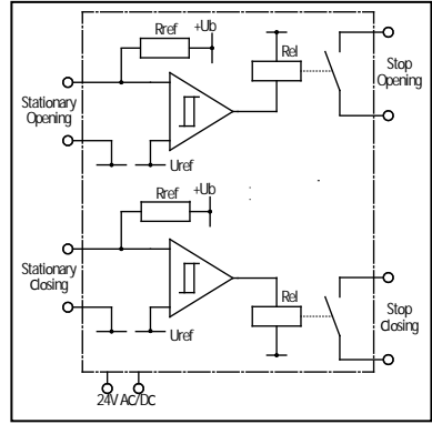
Principeschema SK 32
