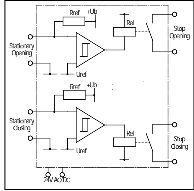
Prinzipialschaltbild SK 32
